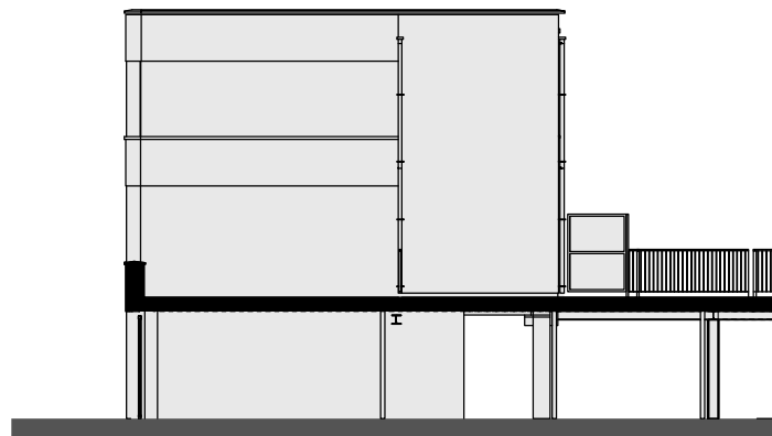
kopgevel bnr. 7
